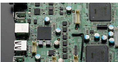
DAC-Board mit digitaler Isolationsschaltung und MMM-Stream-Verarbeitung
